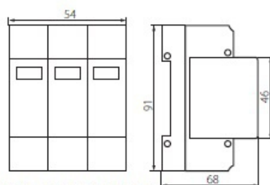
KSD-T1+T2 275/150 3P KSD-T2 275/120 3P
