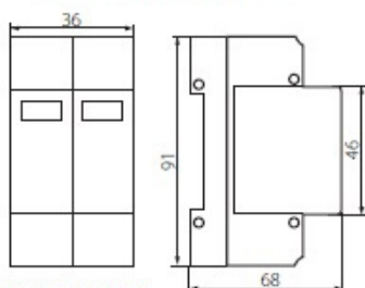
KSD-T1+T2 KSD-T1T2 275/200 3P+N
