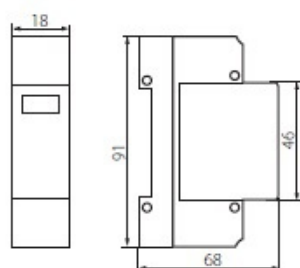
KSD-T2 275/40 1P KSD-T1+T2 275/50 1P
