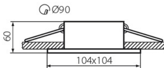
APRILA DTL
