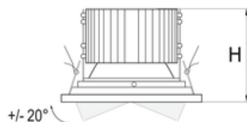
WYCHYLNY \varnothing 135 i \varnothing 160 ADJUSTABLE \varnothing 135 and \varnothing 160
